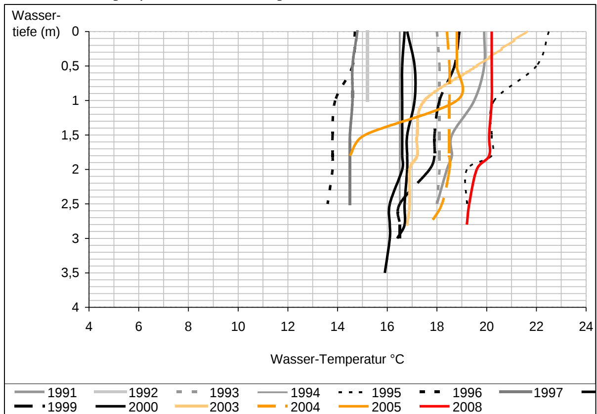
Abb.7: Vertikalprofile der Wassertemperatur im Sommer
