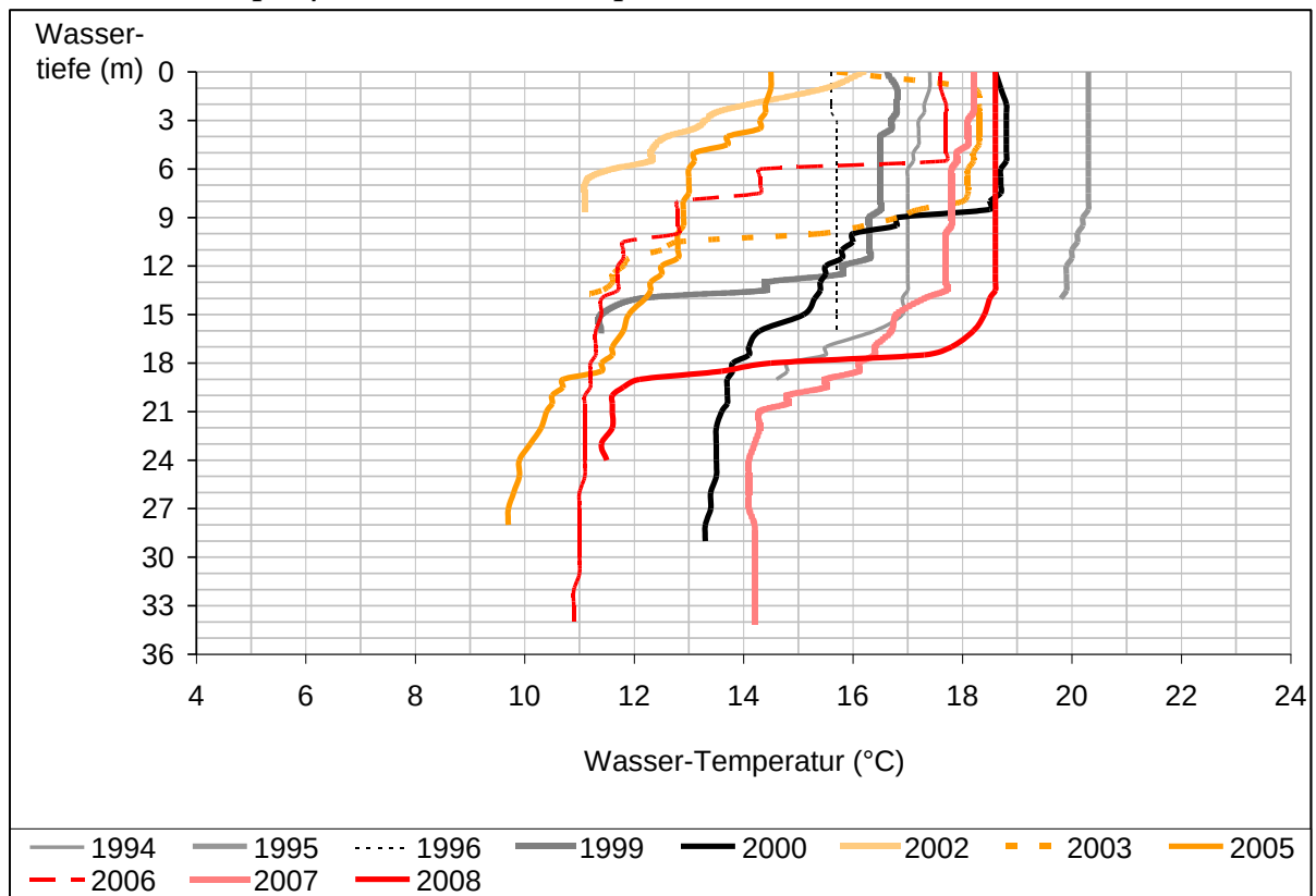
Abb.7: Vertikalprofile der Wassertemperatur im Sommer
