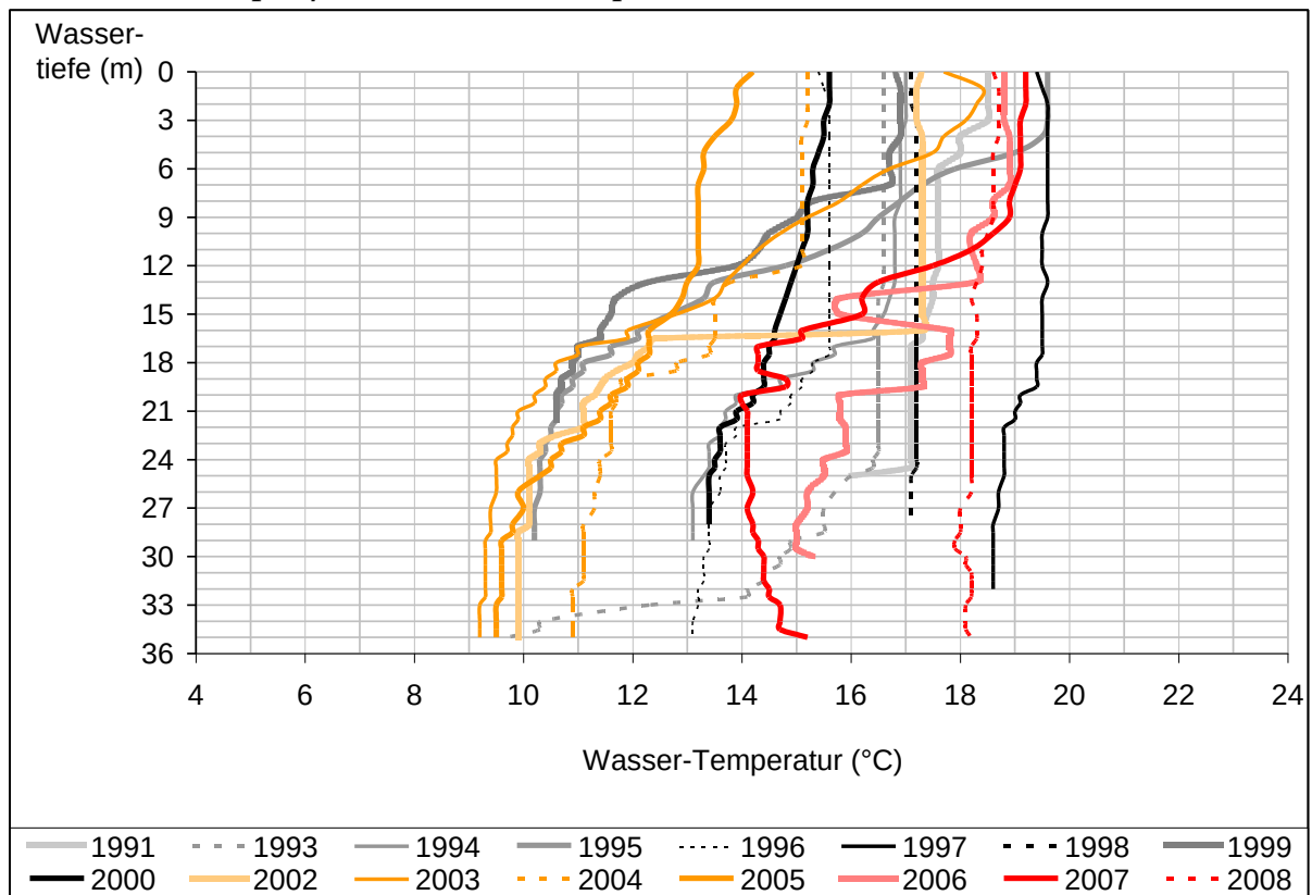
Abb.3: Vertikalprofile der Wassertemperatur im Sommer
