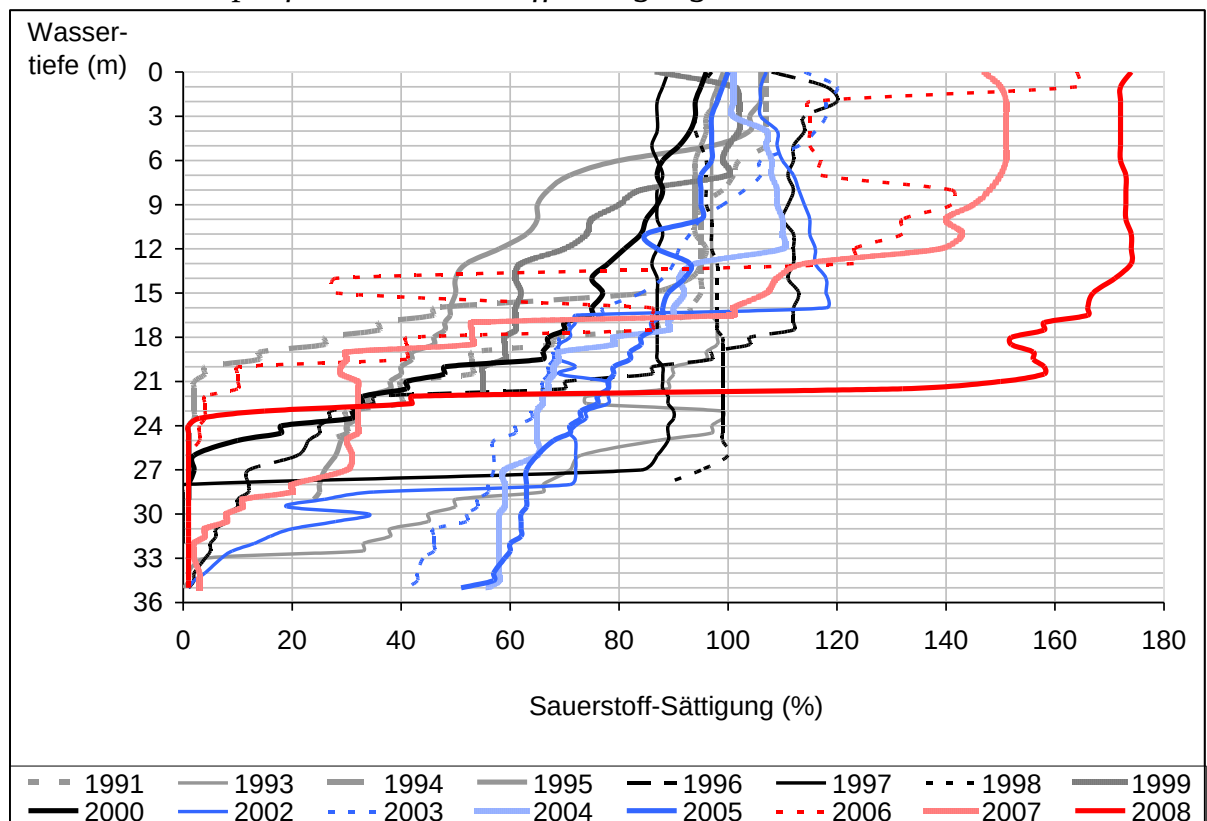
Abb.4: Vertikalprofile der Sauerstoff-Sättigung im Sommer
