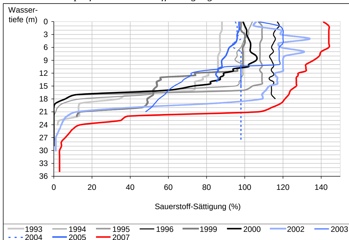
Abb.10: Vertikalprofile der Sauerstoff-Sättigung im Sommer
