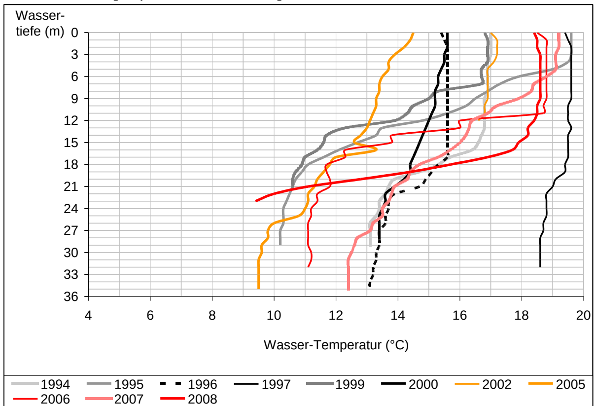
Abb.5: Vertikalprofile der Wassertemperatur im Sommer
