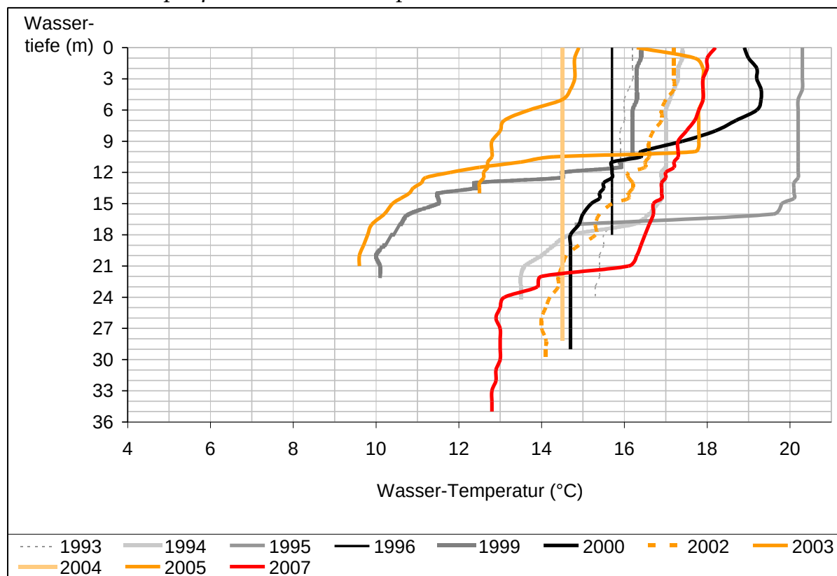
Abb.9: Vertikalprofile der Wassertemperatur im Sommer
