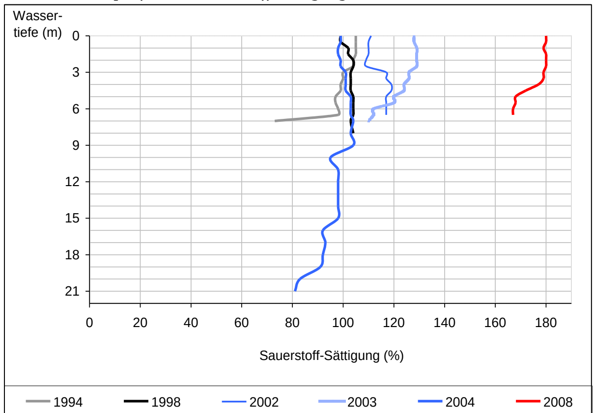
Abb.8: Vertikalprofile der Sauerstoff-Sättigung im Sommer
