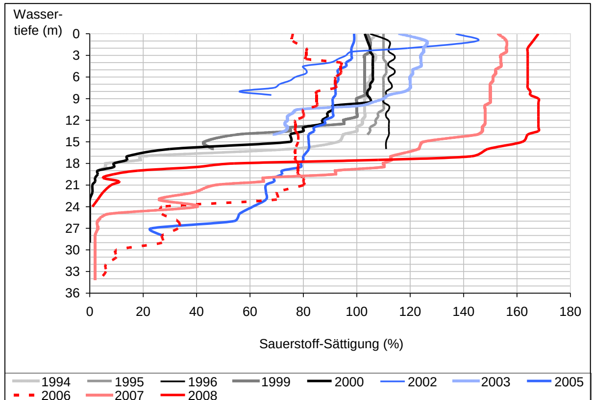
Abb.8: Vertikalprofile der Sauerstoff-Sättigung im Sommer
