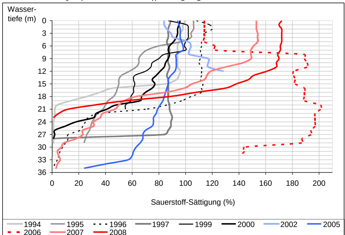
Abb.6: Vertikalprofile der Sauerstoff-Sättigung im Sommer
